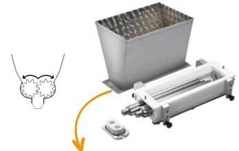
TRÉMIE À CYLINDRE
